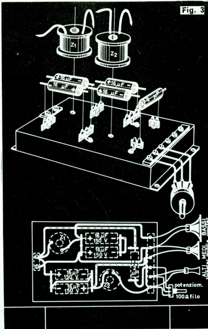
Fig. 3 - Schema di montaggio del filtro.
